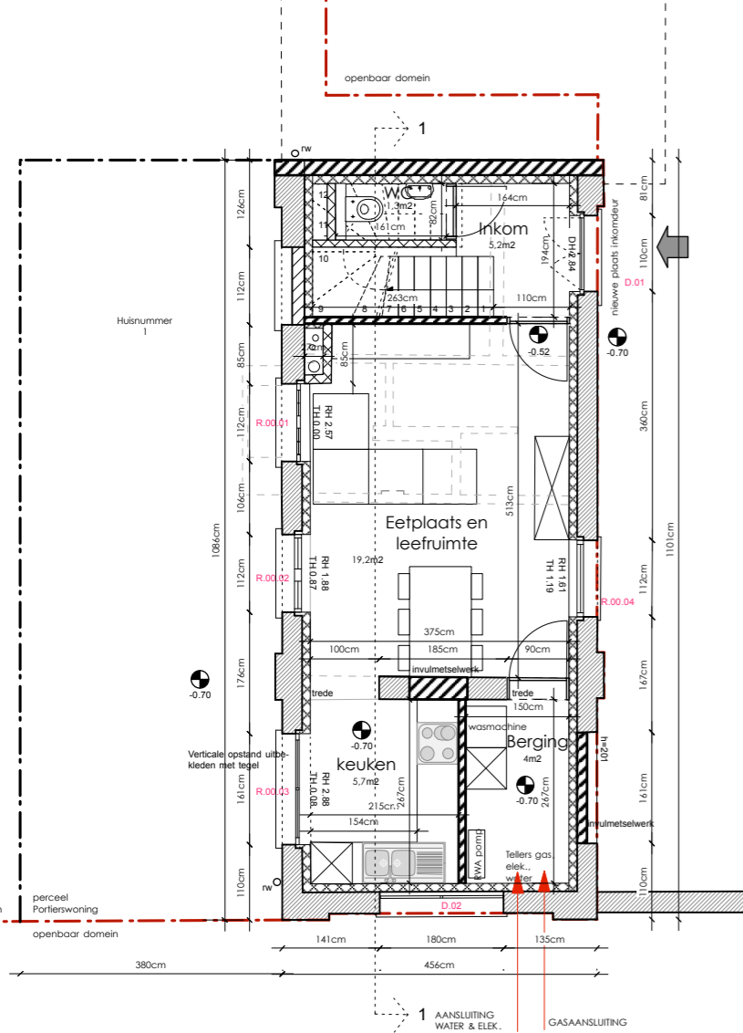
GRONDPLAN
